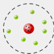
Budowa atomu w modelu Rutherforda (źródło Wikipedia)
